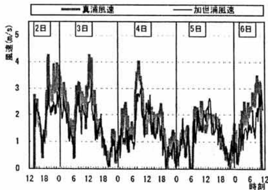
図5 真浦・加世浦における風速
