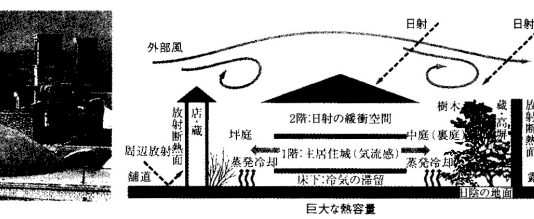
植栽や水面を有して低温面を形成する二つの中庭の空間ボリュームの違いによって生じる圧力差を利用し、室内に風を発生させ、深い軒庇、葺や高層によって日射を遮蔽している京都の町家。 10)
