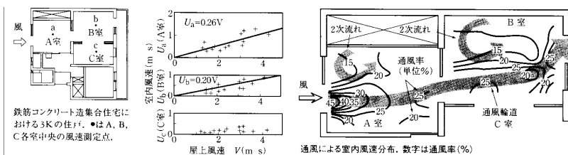
鉄筋コンクリート造集合住宅における3Kの住戸。●はA, B, C各室中央の風速測定点。 屋上風速 V (m/s) と室内風速 U (m/s) の関係 通風による室内風速分布。数字は通風率 (%)
