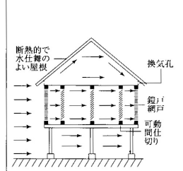
高温多湿地域の開放的な住居。風上と風下で大きな開口を設ける。
