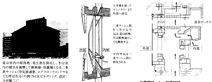
夏は室内の取得熱・発生熱を排出し、冬は室内の暖気を循環して断熱層・防露層となる二重窓サッシ(空気流通窓, エアフローウィンドウなどと呼ばれる)の例(NRCビルディング, 設計: 吉村順三) 二重窓サッシ断面詳細
