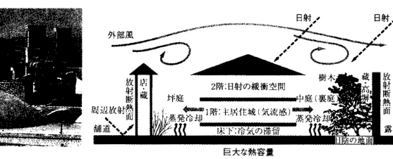
植栽や水面を有して低温面を形成する二つの中庭の空間ボリュームの違いによって生じる圧力差を利用し、室内に風を発生させ、深い軒庇、蔵や高層によって日射を遮蔽している京都の町家。 03
