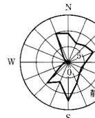
全日の風配
