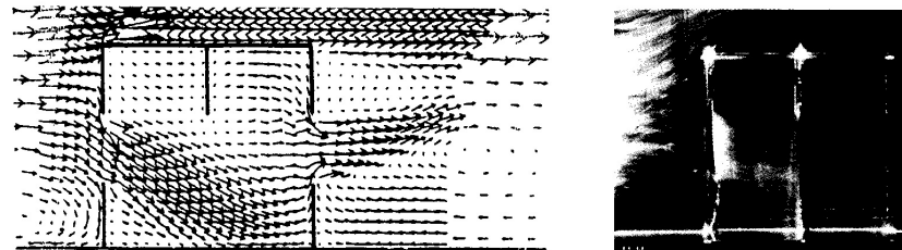
通風の効果は室内の風速分布によっては決定される。間仕切りを有する独立模型内の通風時風速の断面内分布に、乱流数値シミュレーションによる風速ベクトル分布と風洞模型実験により可視化したものを比較すると、両者の気流パターンはよく一致している。
