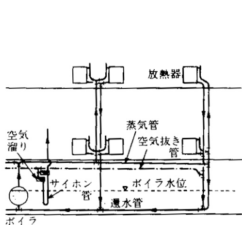
図 ケルチング式蒸気暖房 (参考文献 [3], p. 66)
