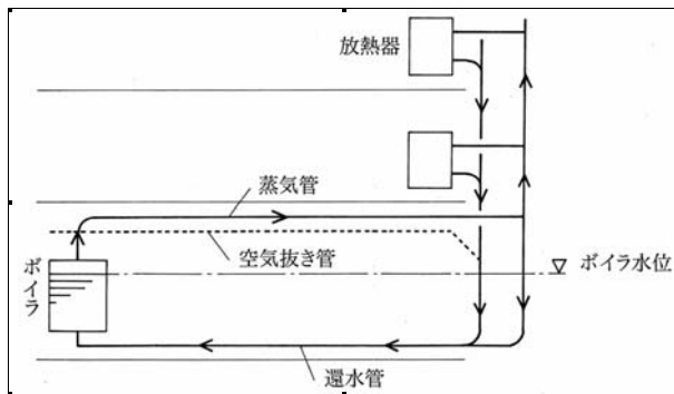
ケルチング式蒸気暖房の模式図 (参考文献 [32], p. 11)
