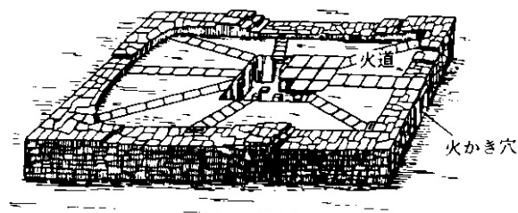
図 溝式床下暖房概略図 (参考文献 [3], p. 3)
