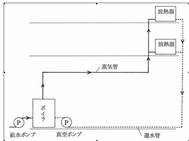
図 ウェブスター式蒸気暖房の模式図 (参考文献 [32], p. 11)
