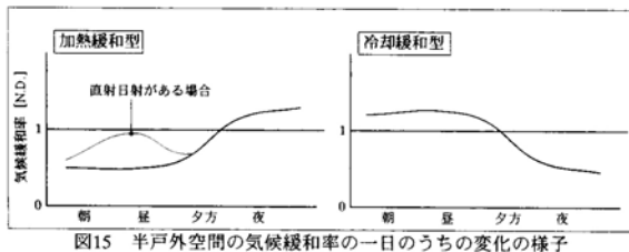
図15 半戶外空間の気候緩和率の一日のうちの变化の様子
