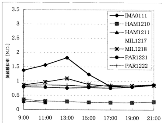
図21 各地の冷却緩和型半戶外空間（冬季）の気候緩和率
